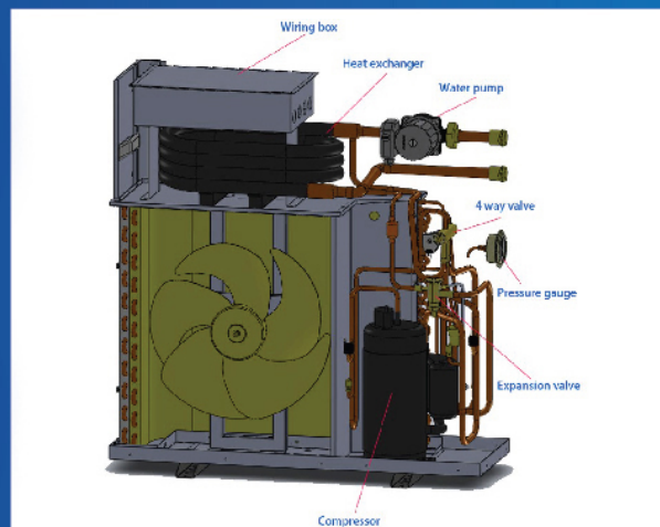
Cấu tạo Heatpump có bơm cho gia đình
